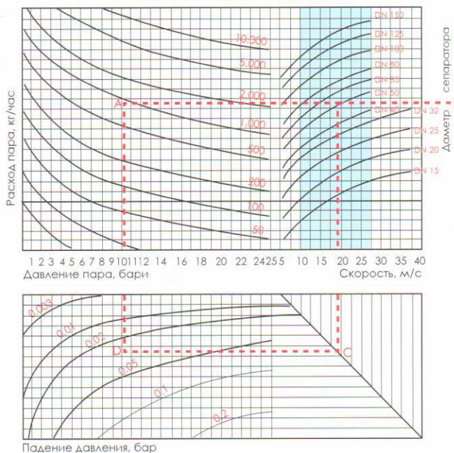
Диаграмма подбора сепаратора
