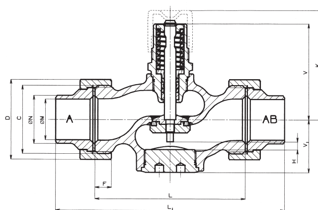
Клапаны RV 111/W с приварным резьбовым соединением
