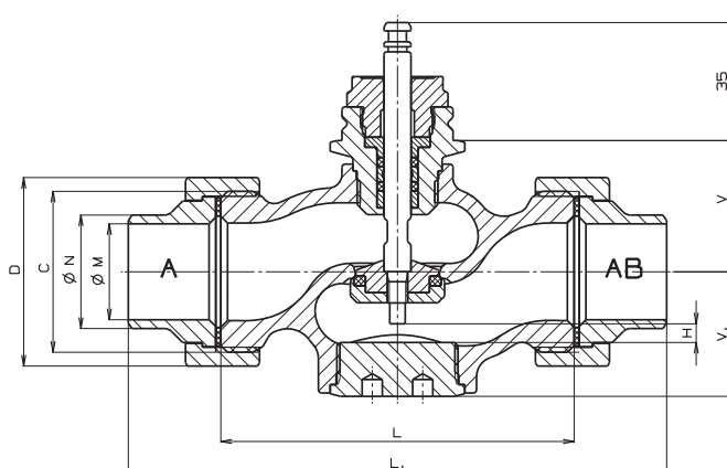
Клапаны RV 111 S/W с приварным резьбовым соединением
