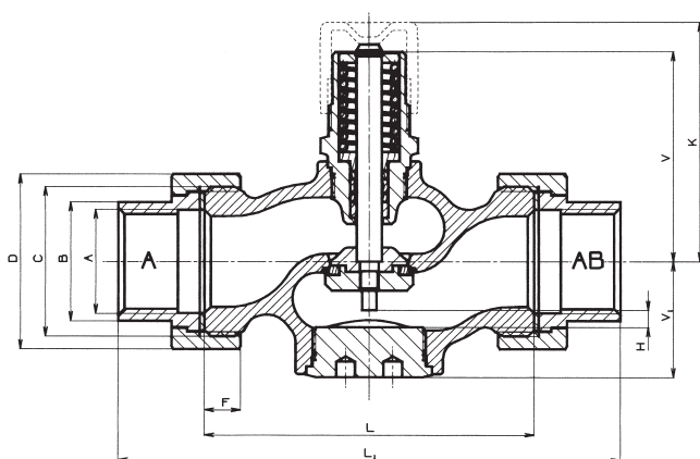
Клапаны RV 111/T с винтовым резьбовым соединением
