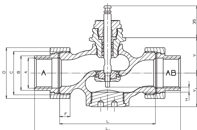
Клапаны RV 111 S/T с винтовым резьбовым соединением
